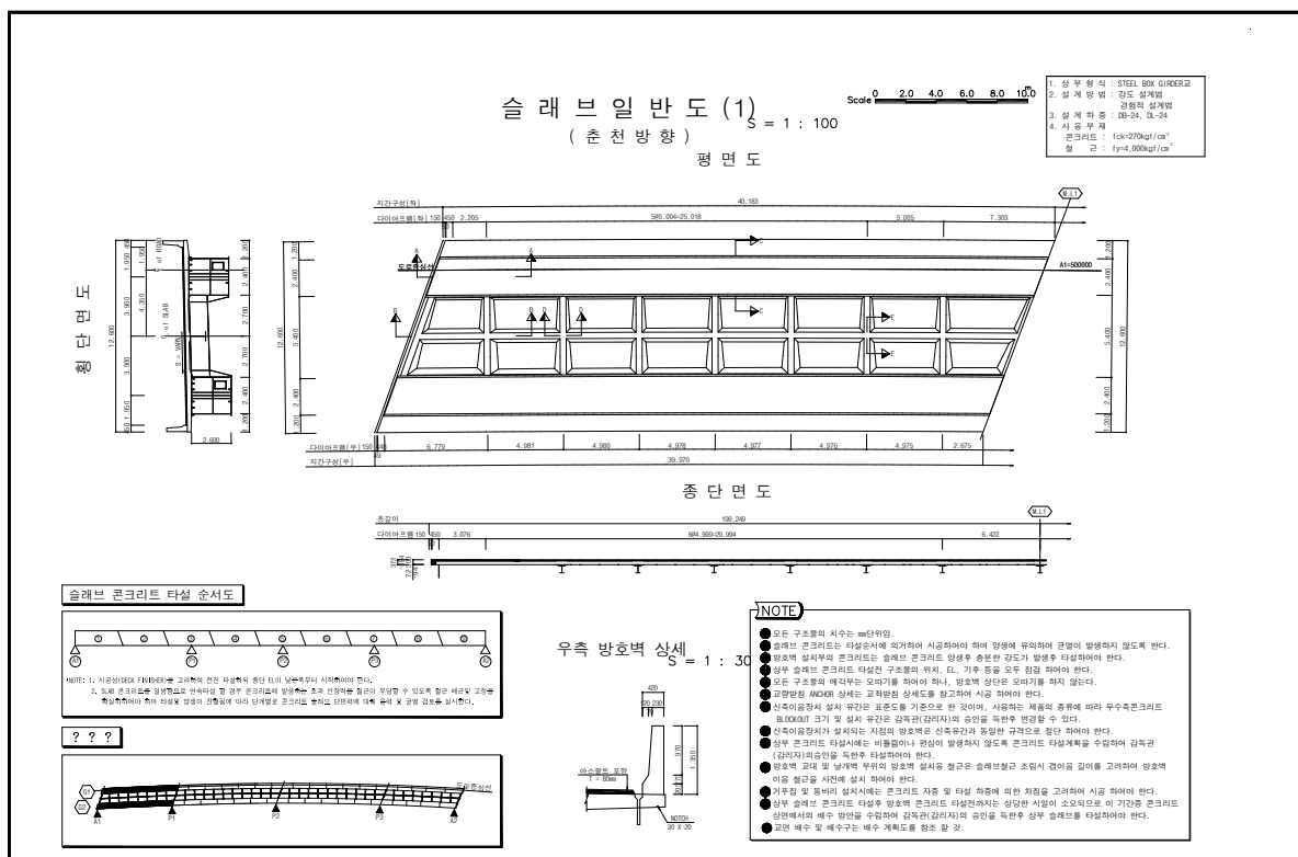
【그림 1.6】 군자4교(양양) 슬래브 일반도
