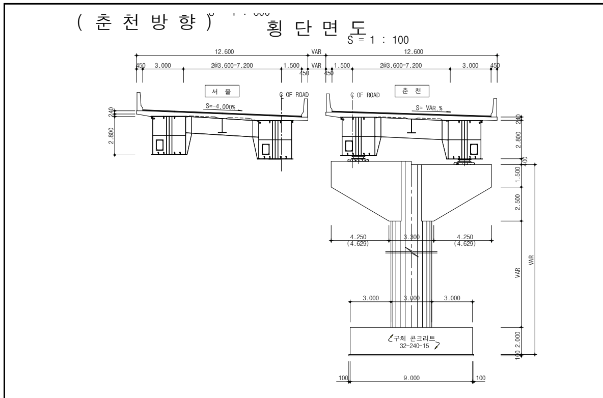
【그림 1.3】 군자4교(양양) 횡단면도
