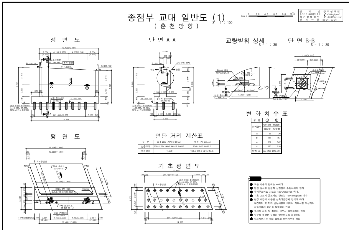
【그림 1.5】 군자4교(양양) 종점교대 일반도
