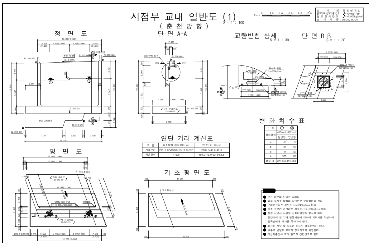
【그림 1.4】 군자4교(양양) 시점교대 일반도
